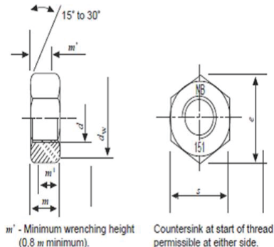
HEXAGON NUTS
